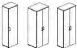
Гардероб O.GB-1 (L)/(R) 560x420x1977 мм O.GB-2 800x600x1977 мм O.GB-4 800x420x1977 мм
