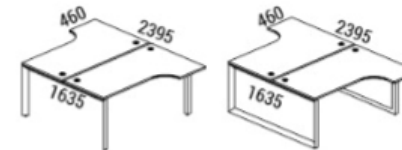
Рабочая станция на П-образном и О-образном м/к
