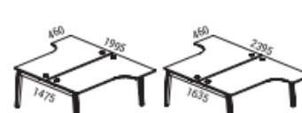
Рабочая станция, опоры - массив дерева
