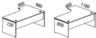
Стол эргономичный левый/правый
